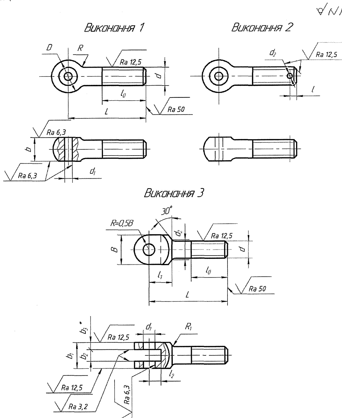
Рисунок 1 – Конструкція болтів
